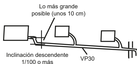
Figura 24 Descarga de agua centralizada
